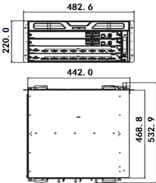
DMC8000-5U
